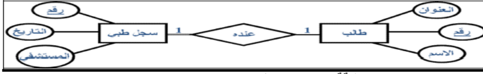
علاقة ١:١ واحد-إلى-واحد (one-to-one)
