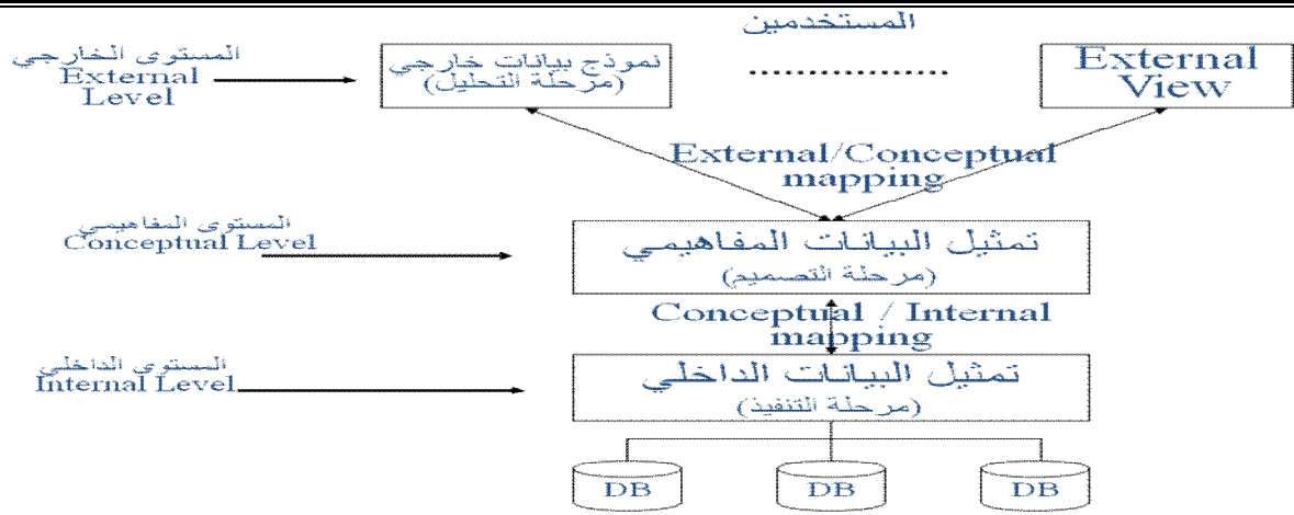
شكل يوضح الثلاث مستويات لمخططات قواعد البيانات (The Three-Schema Architecture)
